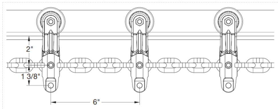
Cadena para Pista en T con TROLLE cada 6"
